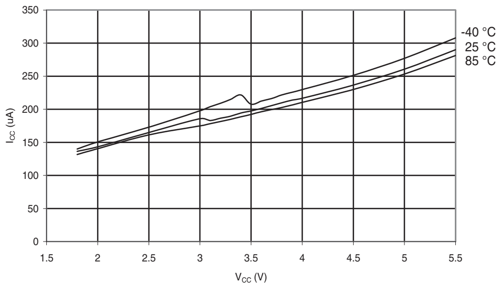
Figure 29-40. ATmega48A: ADC Current vs. V CC (AREF = AV CC )
